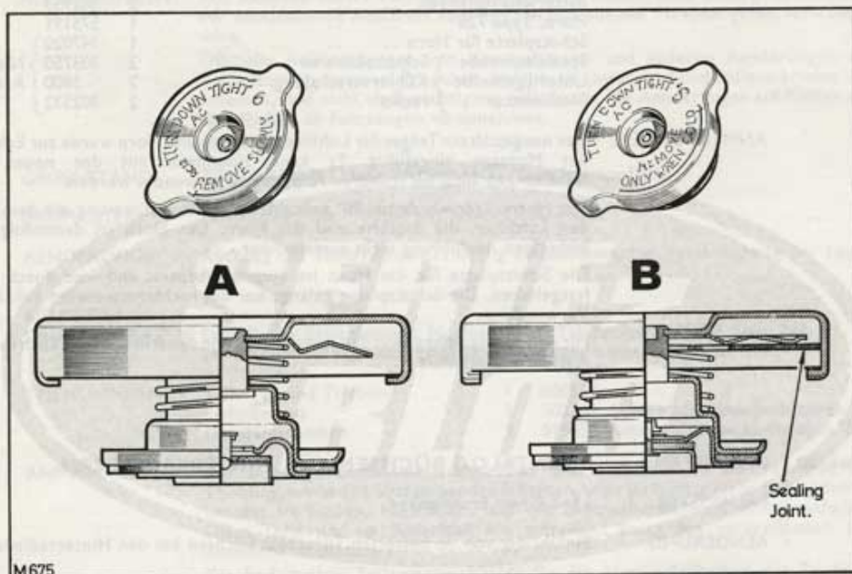
Abb 1. Unterscheidungsmerkmale der Kühlerdeckel
